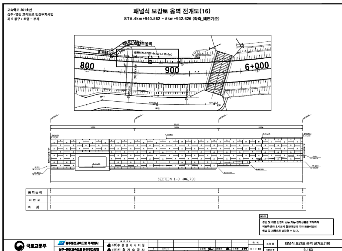
【그림 8.4】 전개도(계속)
