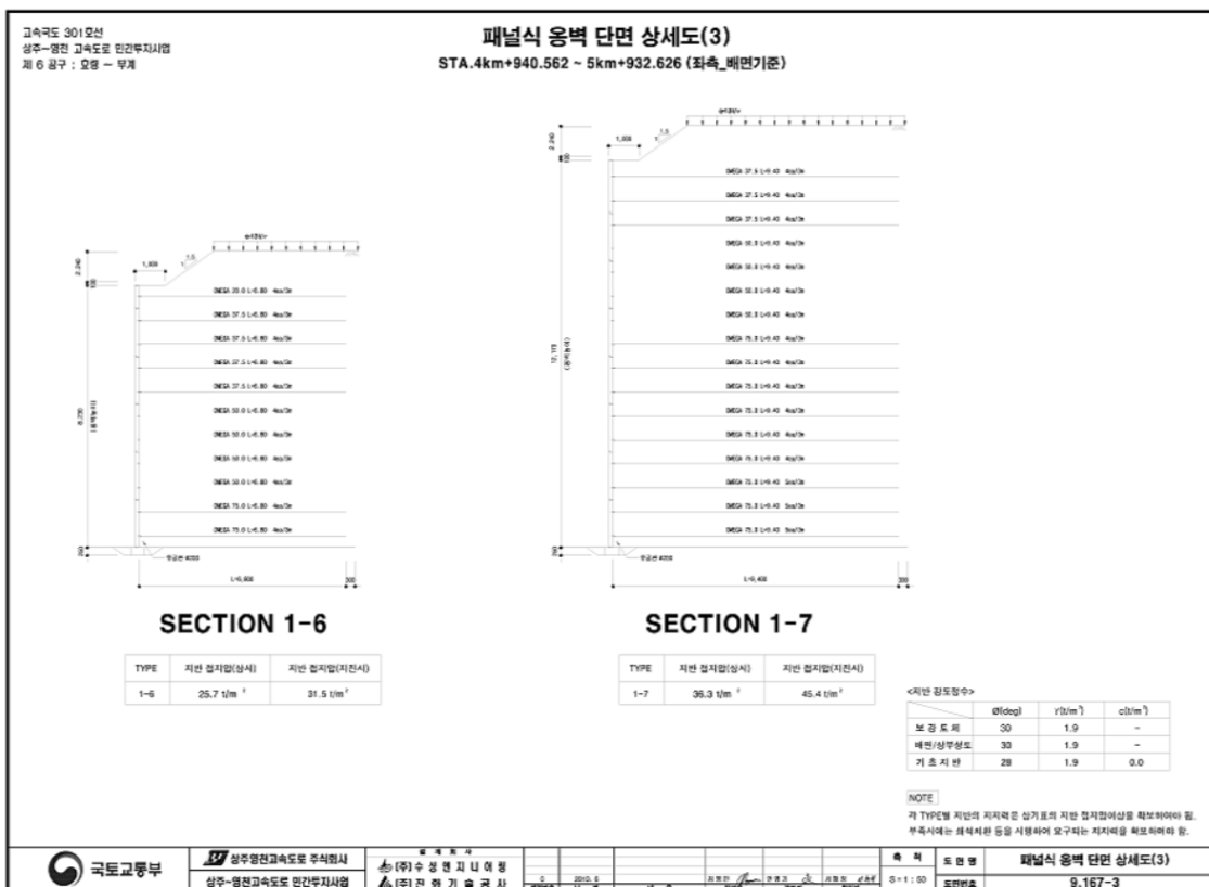
【그림 8.5】 단면도(계속)
