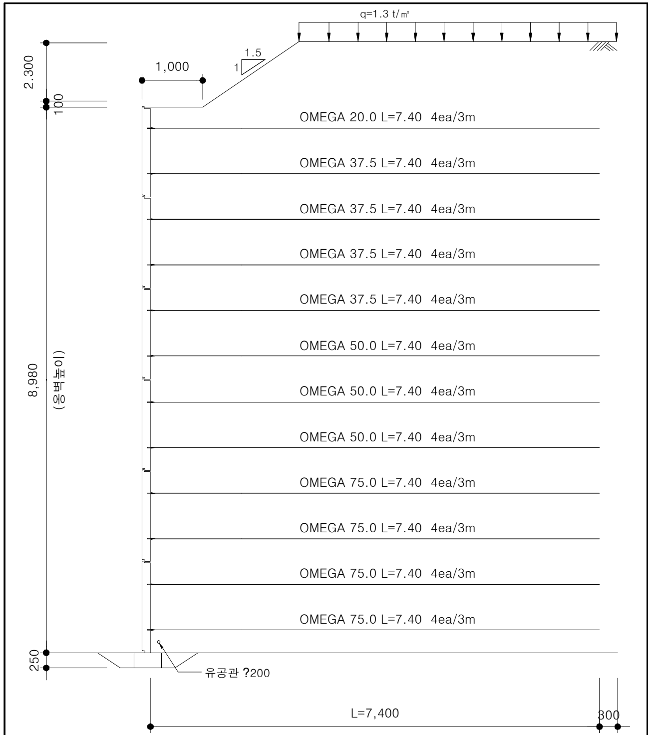
【그림 74.10】 검토단면도
