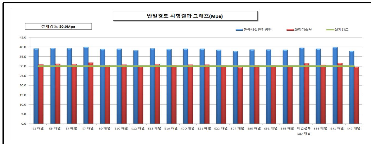
【그림 74.7】 【그림 1.4.2】반발경도시험 측정결과
