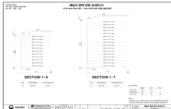
단면도
