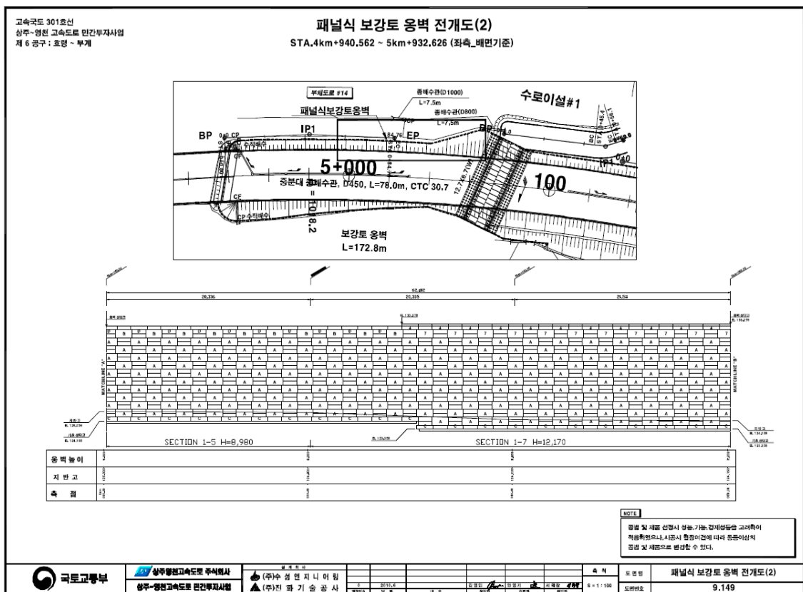
【그림 74.4】 전개도
